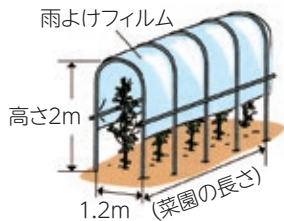
図3 雨よけ
