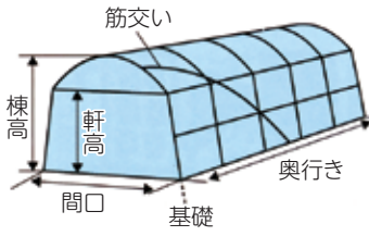
図1 ハウスの構造
