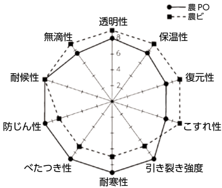
図2 農ビと農POの性能比較
